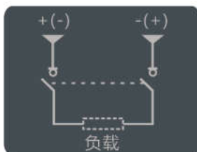
2 极串接线图 (DC1000V)
