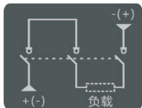
3 极串接线图 (DC1500V)
