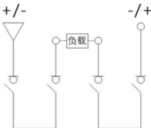
接线图 1 4P 外形 C 型接线方式
