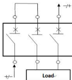
三极串 接线图
