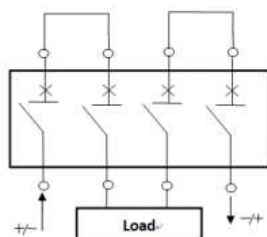
四极串 接线图
