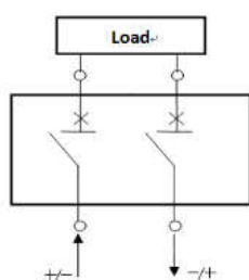
二极串 接线图
