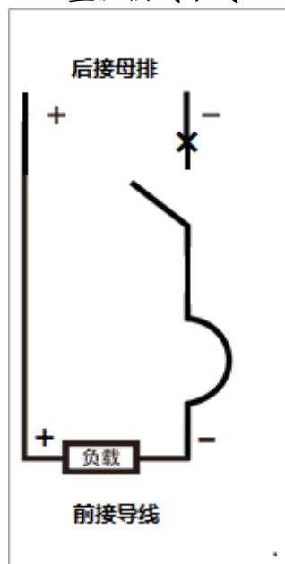
直流接线方式
