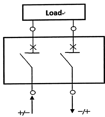
二极串 接线图
