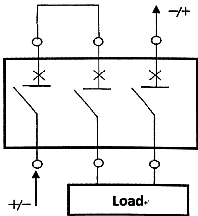
三极串 接线图
