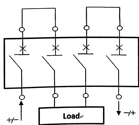
四极串 接线图
