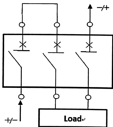
三极串 接线图
