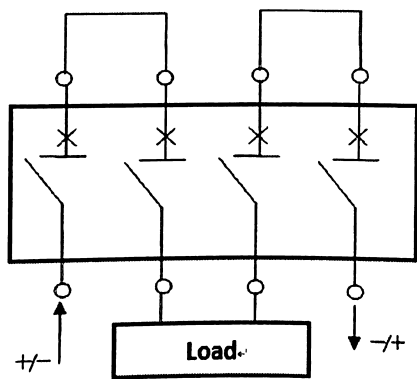
四极串 接线图
