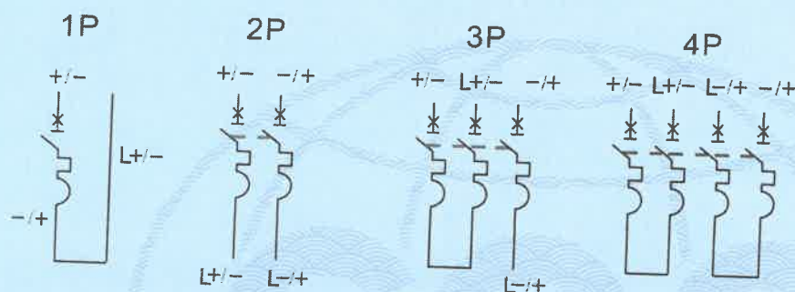
TGB1Z-125直流线路接线图
