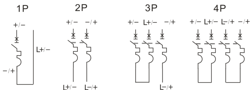
TGB1Z-125直流线路接线图
